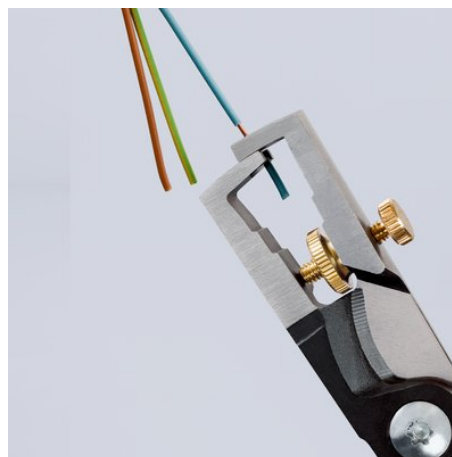
Lengdemarkering: Optiske markeringer understøtter ved gjentatt avisolering av like lengder (11 mm og 16 mm)
